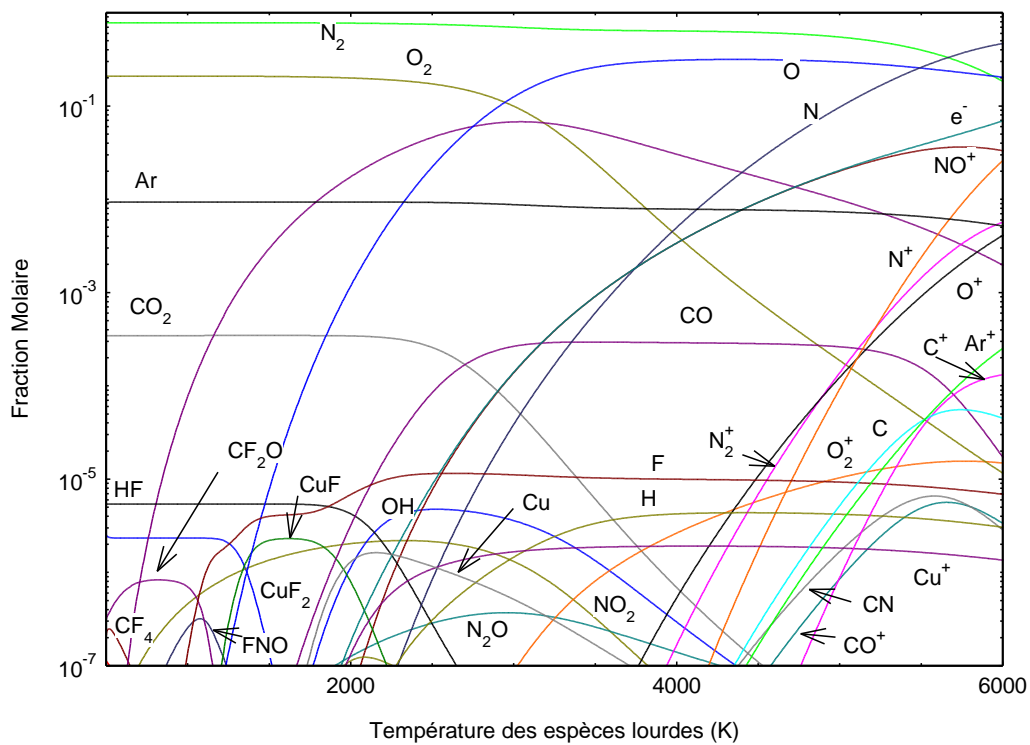
Figure 6.c: Fraction molaire du mélange 3 (1,95 g air sec, 0,01 g cuivre, 0,02 g PTFE, 6 \times 10^{-6} g vapeur sèche) à la pression de 10^5 Pa et avec un déséquilibre thermique ( \theta = T_e/T_1 ) de 2.
