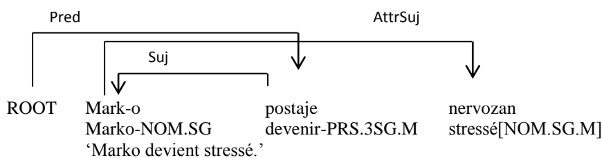
Exemple 2: Etiquette AttrSuj
