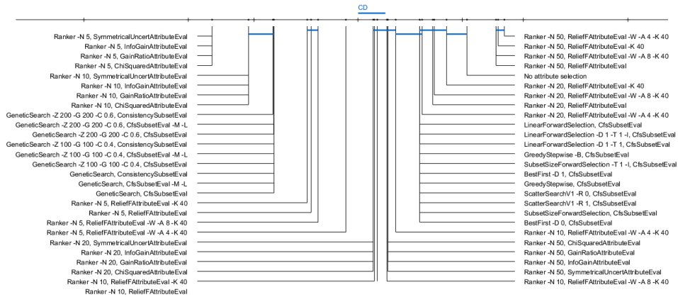
FIG. 1 – Résultats du test de Nemenyi sur les méthodes de sélections d'attributs employées au méta-niveau. Les méthodes sont classées par performance croissante et les groupes connectés ne sont pas jugés significativement différents.
