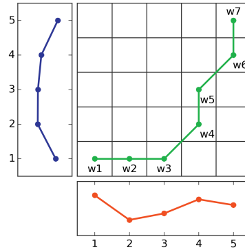
(d) DTW warping path
