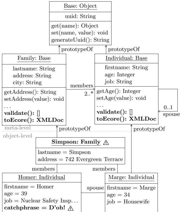
Fig. 3: FlexiMeta Code Generator
