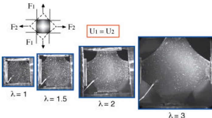
Figure 3. Principe de l'essai de traction simultanée
