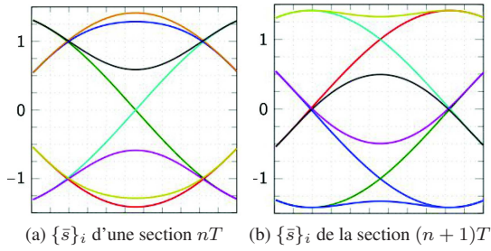
FIGURE 3: Banc de filtres exact pour une L=2 , REC, h=3/4
