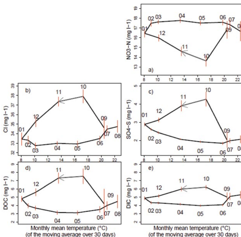
Figure 3 : Moyennes mensuelles des concentrations en (a) nitrate-N, (b) chlorure, (c) sulfate-S, (d) COD et (e) DIC (mg.l -1 ) en fonction des moyennes mensuelles des moyennes glissantes sur une fenêtre de 30 jours des températures. L’hystérèse est horaire pour le nitrate, anti-horaire pour les autres solutés. Les barres d’erreur représentent les intervalles de confiance [Aubert et al., 2013b].
