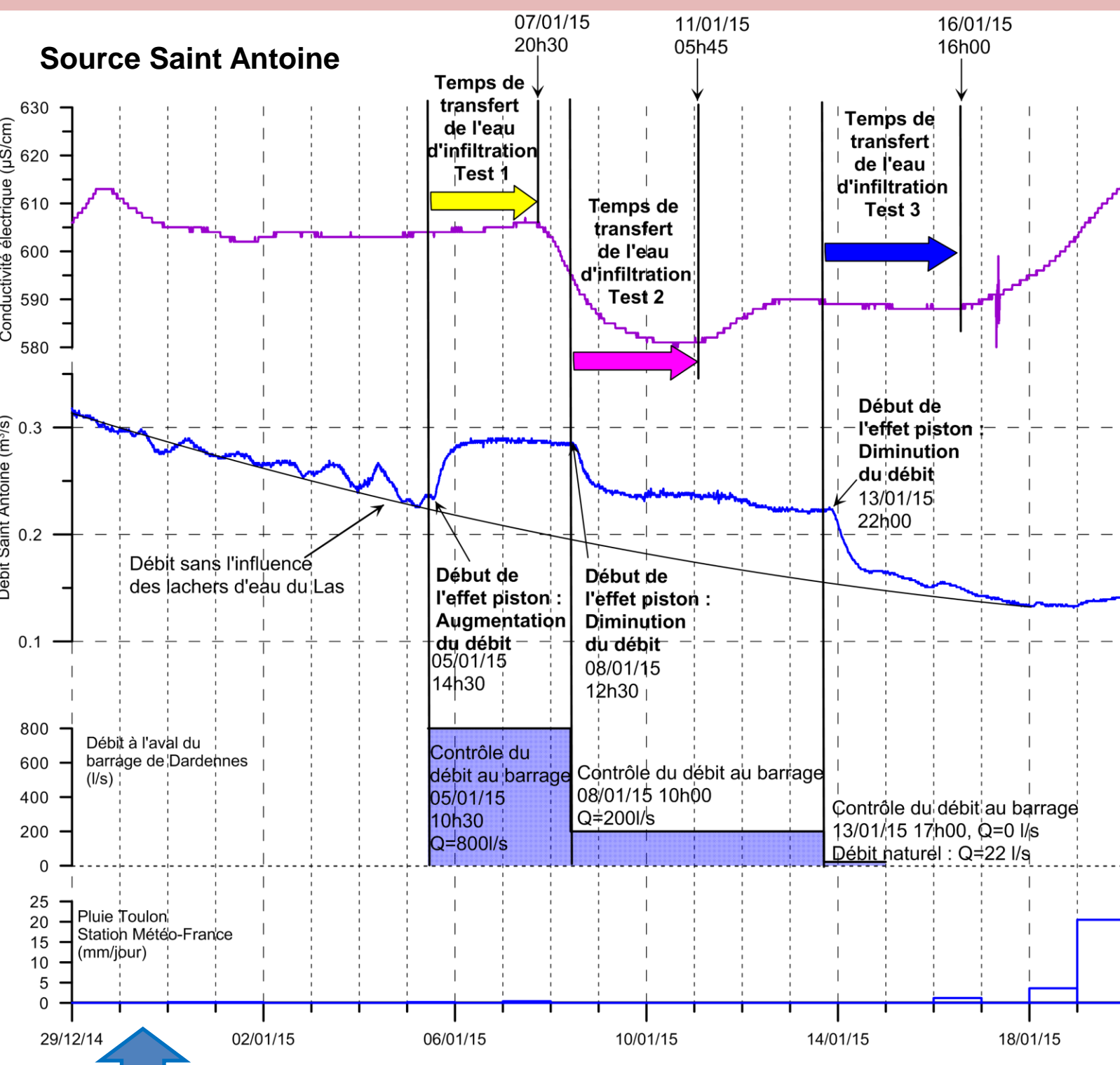
Figure 5 : Evolution de la conductivité électrique et du débit de la source Saint Antoine durant les tests hydrauliques. Les légendes sur le graphique montrent le temps de décalage entre la variation de débit dans le Las et l'arrivée de l'onde de pression (effet piston). Les flèches horizontales montrent le temps de transfert entre l'eau dans le Las et la première arrivée de l'eau d'infiltration jusqu'à la source qui est marquée par la variation de conductivité électrique.
