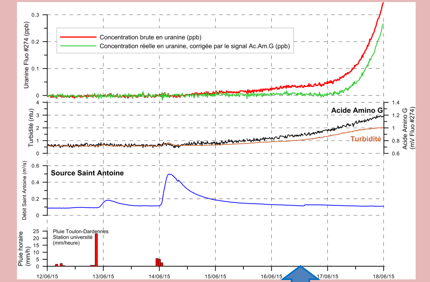
Figure 7 : Concentration en uranne brute (correction sur la turbidité uniquement) et réelle avec une correction supplémentaire utilisant le signal de l'Acide Amino G du fluorimètre (GGUN Cat. 3) représentatif de la fluorescence de la Matière Organique variable en fonction des crues.
