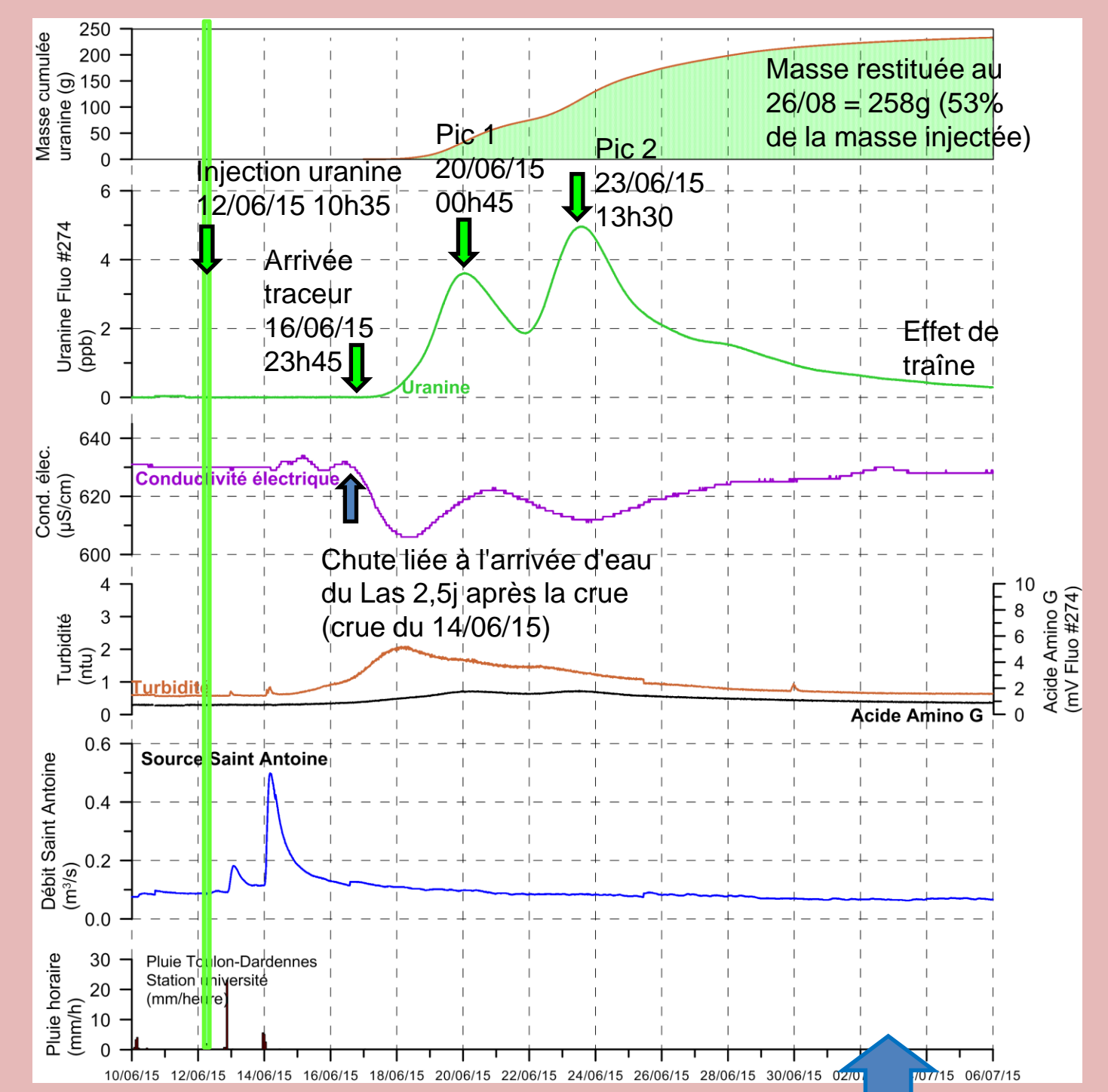
Figure 6 : Evolution au cours du temps des mesures CTD et du fluorimètre GGUN au pas de temps de 15 minutes sur la source Saint Antoine lors du traçage artificiel du 12/06/2015 à la perte du Las au hameau de Dardennes.
