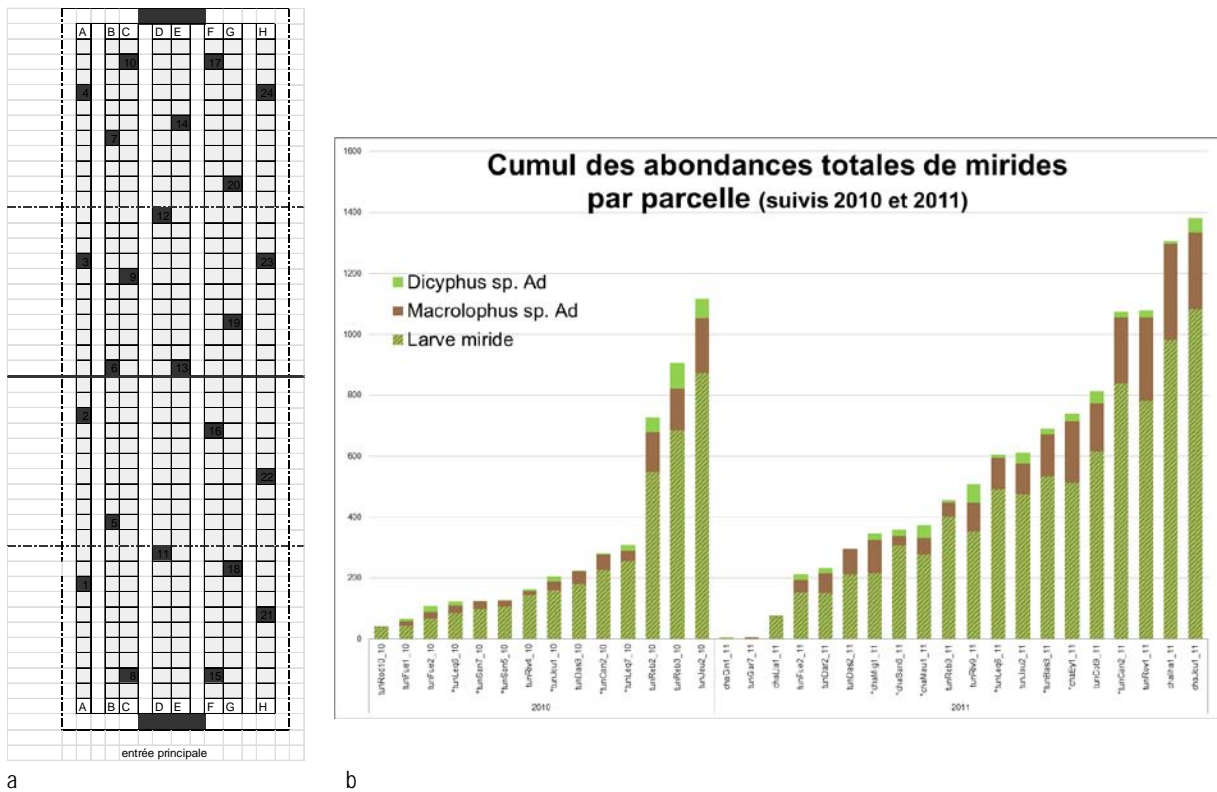
Figure 1 : a- schéma de tunnel : repérage des 24 zones d'observation ; b- résultat obtenu : abondances des mirides par parcelle.
