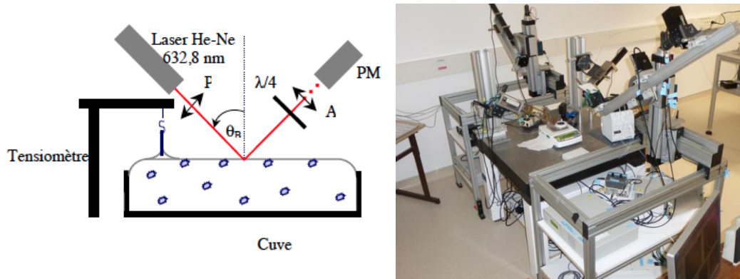
Figure 2. Schéma de principe de l'ellipsomètre à annulation à l'interface eau-air : l'angle d'incidence est égal à l'angle de Brewster - 1^\circ (soit 52.01^\circ )
