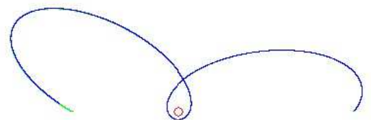
Orbite au voisinage de l'horizon (cercle rouge) d'un trou noir
