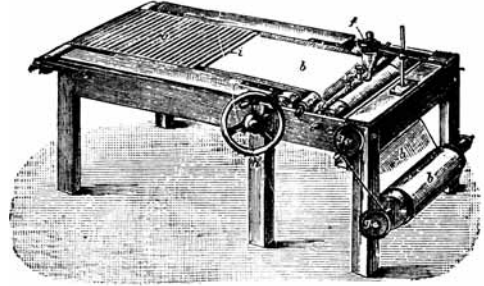
Hình 101 Những máy được sử dụng trong việc chế tạo giấy in ra ảnh POP, hình chạm khắc, khoảng 1890.
