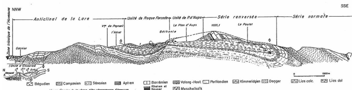
Fig.96. - Coupe de la Sainte-Baume par le Plan d'Aups. (d'après J.P.H. Caron, G. Guieu, C. Templar, légèrement modifié pour l'unité de Roqueforcade à la suite d'un forage exécuté en S (1970) car le Lias chevauchant s'est révélé être encore plus mince que prévu).
