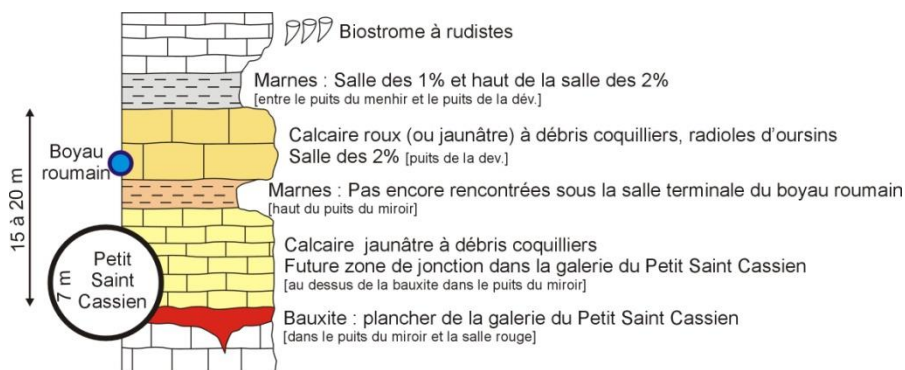
Figure 7 : Log géologique représentant les différentes strates observées dans la première partie de l'Eau-Relie et qui se retrouvent décalées 95 mètres plus bas dans le fond du gouffre (extrait de Arfib et Seurin, 2013).
