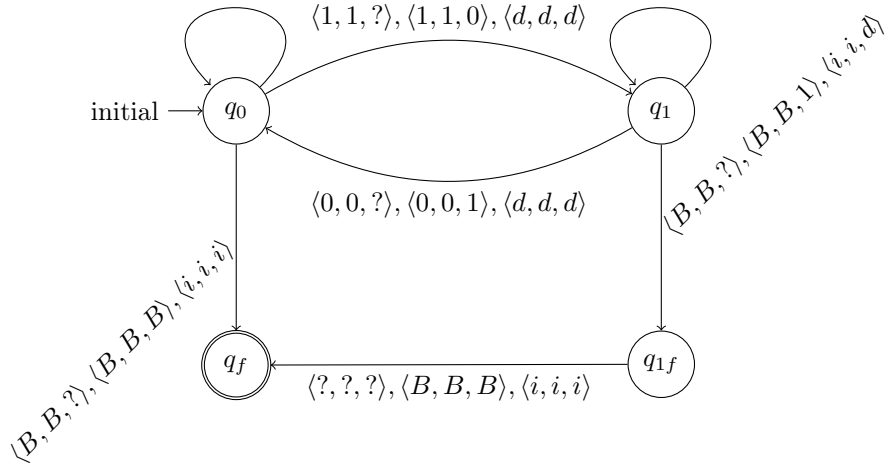
FIGURE 1 – Une machine de Turing sur l’alphabet \{0, 1, B\} , à 3 rubans, qui met sur la troisième bande le résultat de l’addition des nombres écrits en binaire sur les deux premières, chaque nombre étant écrit de la gauche vers la droite à partir de la position initiale de la tête sur ce ruban et suivi d’un B . À la fin du calcul, les têtes sont sur les B finaux des trois nombres. L’état final est entouré d’un double trait. Une transition dénotée \langle l_1, l_2, l_3 \rangle, \langle e_1, e_2, e_3 \rangle, \langle d_1, d_2, d_3 \rangle s’interprète ainsi : si les cases sous les têtes de lectures sont étiquetées l_1, l_2, l_3 alors la machine écrit sur ces cases e_1, e_2, e_3 puis chaque tête numéro i fait le pas dicté par d_i , i dénotant l’immobilité et d le mouvement vers la droite. Par souci de compacité, on note ? pour signifier que la valeur lue n’importe pas : une telle transition est une abréviation pour plusieurs transitions obtenues en remplaçant ? par 0, 1, B . L’état q_0 (resp. q_1 ) dénote l’absence (resp. la présence) de retenue entrante, l’état q_f est final, et l’état q_{1,f} sert à écrire un B final sur la troisième bande une fois qu’on y a écrit comme chiffre le plus significatif un 1 issu d’une retenue.
