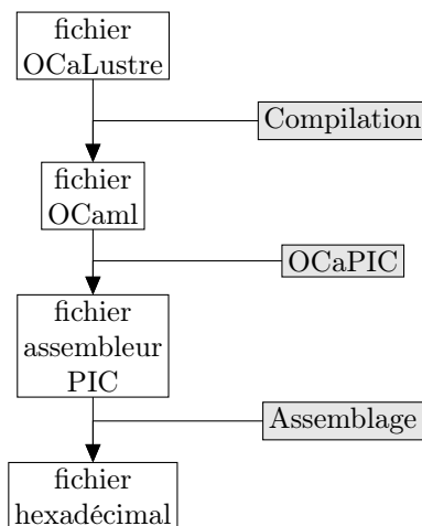
FIGURE 2 – Chaîne de compilation d'OCaLustre pour microcontrôleurs PIC
