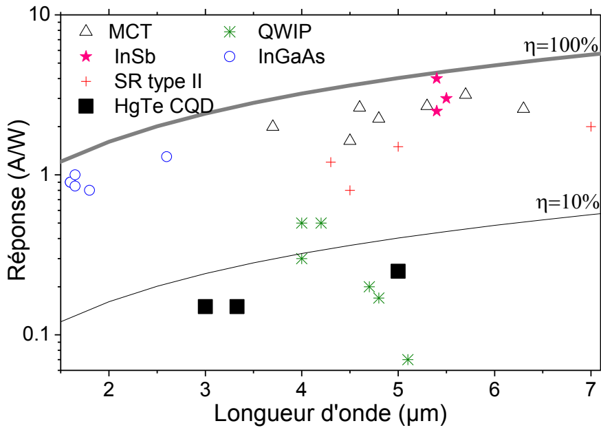
Figure 6 : Réponse de détecteur issu de différentes technologies en fonction de leur longueur d'onde de détection
