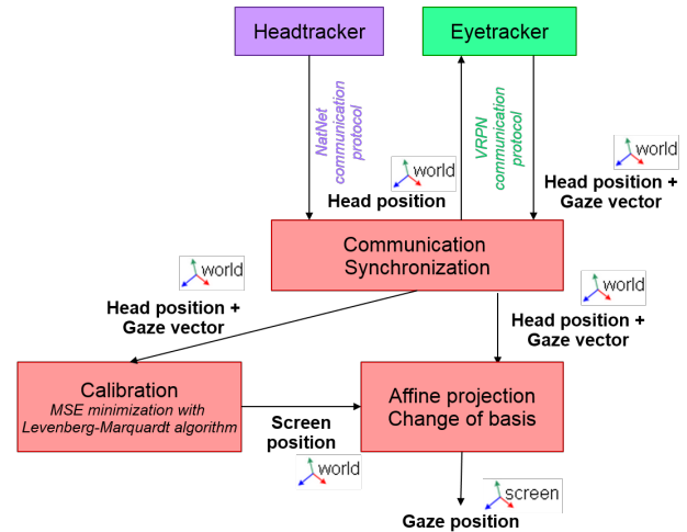
(a) EHT operating scheme.
