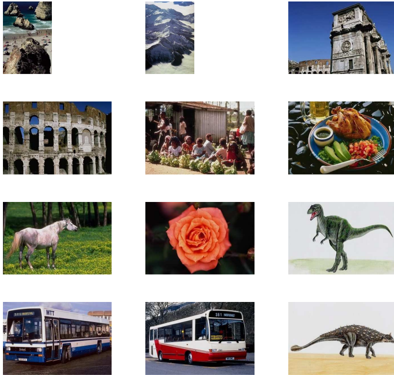
Fig. 13. SIMPLicity Dataset
