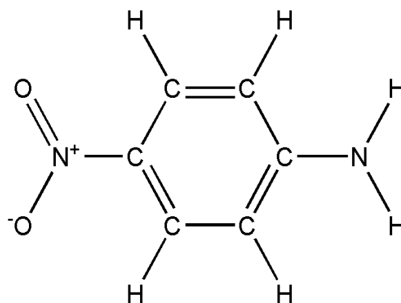
p -Nitroaniline
