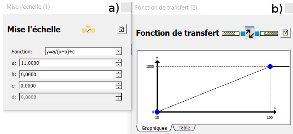
FIGURE 5 – a) Conversion tension en distance (distance = a/tension); b) fonction de transfert entre distance (abscisses en mm) et vitesse d'avance du robot (ordonnées en mm/s)
