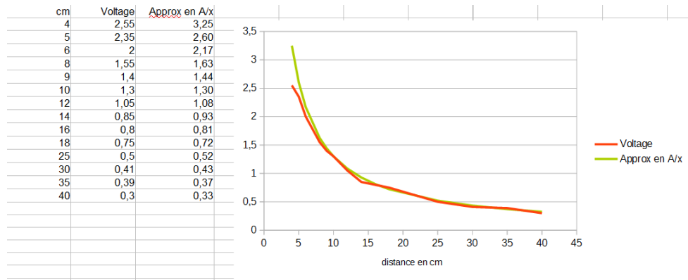
FIGURE 4 – Calibration et modélisation d'un capteur de distances à infrarouge.
