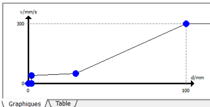
FIGURE 3 – Exemple d'une rampe de vitesse à l'approche d'une pose. En abscisse la distance à la pose en mm ; en ordonnée la vitesse d'avance du robot en mm/s.
