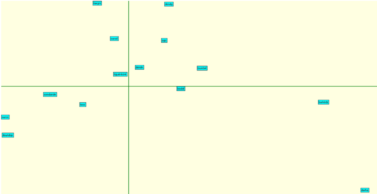
Figure 3 : AFC sur les localités, plan des deux premiers facteurs (tableau des 602 formes les plus fréquentes dans chacune des 14 localités)
