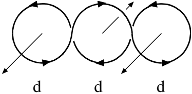
Fig. (1) The Quarks
