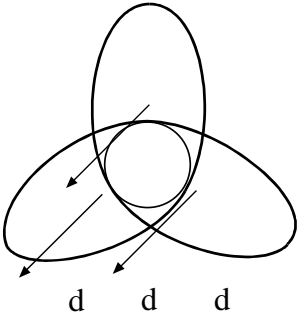
Fig. (2) Quarks
