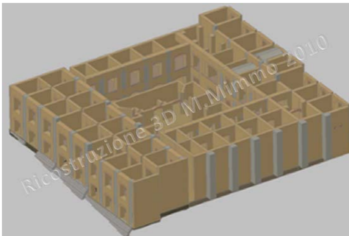
Fig. 7 - Proposta ricostruttiva dell'edificio occidentale degli horrea Vespasiani con vista da NW, privo di copertura.
