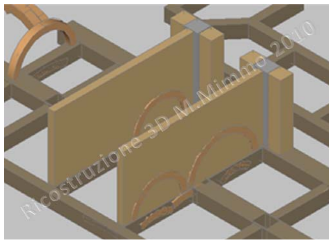
Fig. 10 - Analisi del sistema spingente collocato a livello fondale e d'alzato; restituzione 3d delle stesse strutture.
