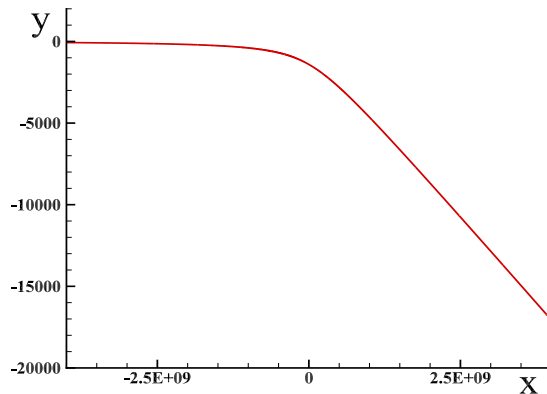
FIGURE 3. Déflexion de la lumière par le champ de gravité solaire, y = y_0 - R
