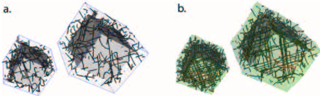
Figure 3 – Evolution des microstructures de dislocation depuis l'état initial (a.) jusqu'à une déformation de \gamma^p = 0.1\% (b.). La densité de dislocation initiale est \approx 2.10^{13} m^{-2} . On notera l'accumulation des dislocations aux interfaces après déformation.
