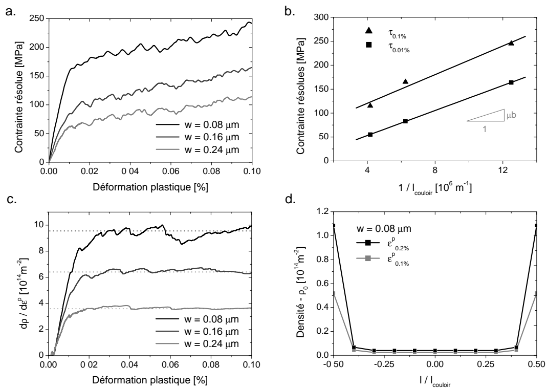
Figure 4 – a. Courbes contrainte résolue (MPa) - déformation plastique (%) pour trois tailles de couloirs de matrice (0.08, 0.16 et 0.24 \mu\text{m} ) avec une fraction volumique identique ( f = 61\% ), b. Courbes contrainte résolue (MPa) en fonction de 1/l_{\text{couloir}} pour \gamma^p = 0.01\% et 0.1\% pour les 4 largeurs de couloir, c. taux de croissance des densités de dislocation en fonction de la déformation plastique, et d. le profil des densités de dislocation dans la matrice pour une taille de couloir de 0.08 \mu\text{m} .
