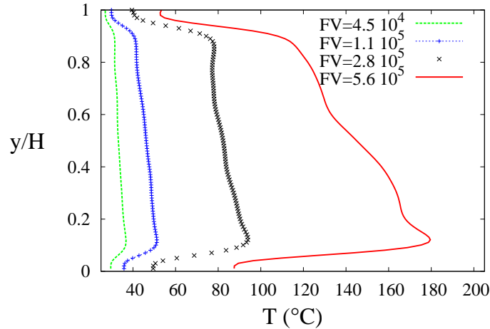
Figure 3 – Profils de température générée ( \mu = 0,3; t = 0,02s ).
