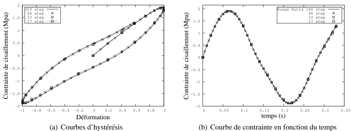
Figure 2 – Test de cisaillement
