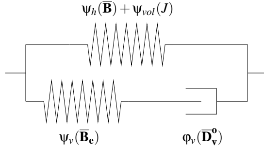
Figure 1 – Modèle de Zener
