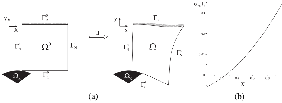
Figure 1 – (a) Domaine initial et déformé avec obstacle rigide, (b) Contrainte normale (\sigma_{nm}J_s) sur le bord \Gamma_C^0 .
