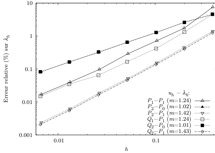
Figure 4 – Erreur relative en norme L^2 ( \|\sigma_{nn}^- J_s - \lambda_h\|_{0,\Gamma_C^0} / \|\sigma_{nn}^- J_s\|_{0,\Gamma_C^0} ) en fonction de la taille des éléments ( h ).
