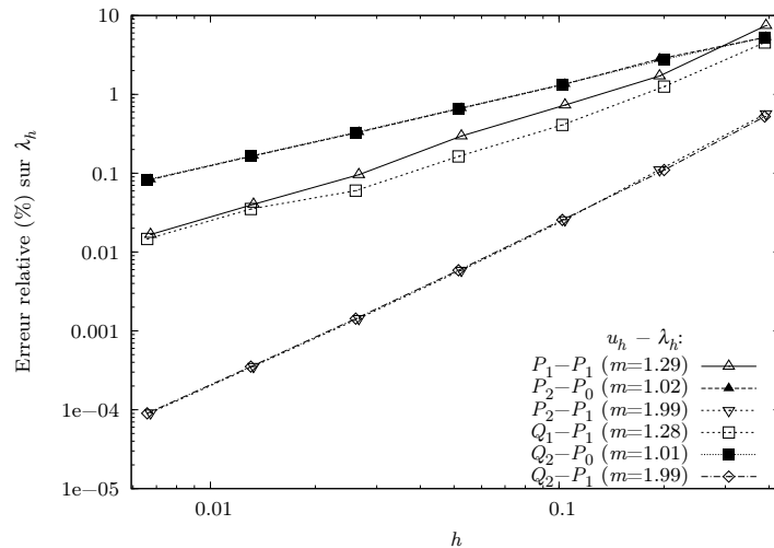
Figure 5 – Erreur relative en norme L^2 ( \|\sigma_{nn}^- J_s - \lambda_h\|_{0,\Gamma_C^0} / \|\sigma_{nn}^- J_s\|_{0,\Gamma_C^0} ) en fonction de la taille des éléments ( h ) pour les maillages dont un sommet est à X = 1/4 .
