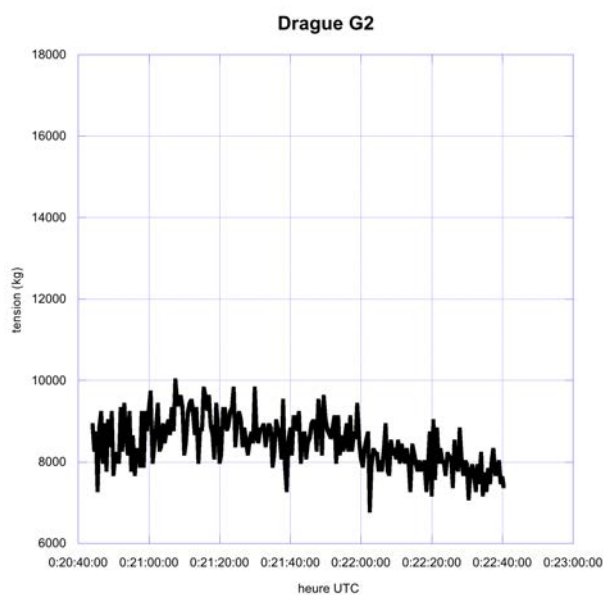
Figure 22: tension du câble pendant le dragage G2
