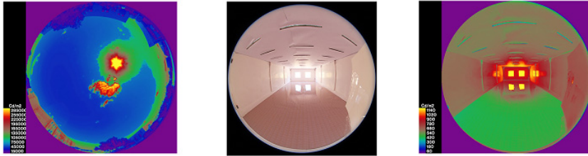
Figure 5. L'ambiance lumineuse intérieure du modèle équipé de Plafond anidolique à 10 h
