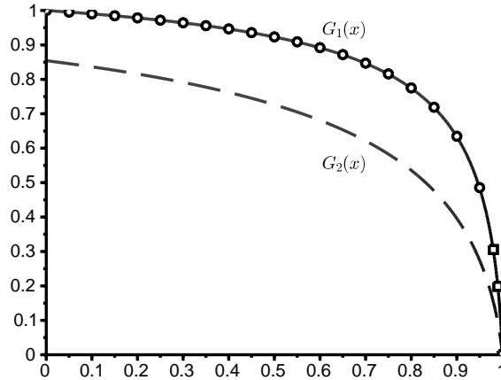
FIGURE 4 – Le cas où a_1 = 3,2 . Comparaison des formules (25) [petits cercles] et (26) [petits carrés] pour G_1(x) avec la fonction génératrice du vecteur propre associé à la valeur propre \mu_N de la matrice tronquée \mathcal{M}^{(N)} (ligne continue) avec N = 10^4 .
