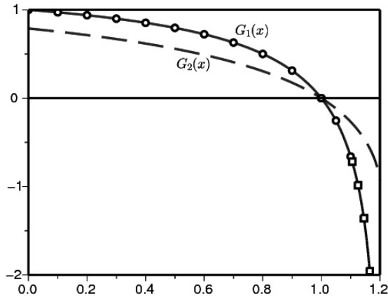
Рисунок 3. Корпус a_1 = 2,5 , Отслеживаем производящие функции G_1(x) (сплошная линия) и G_2(x) (пунктирная линия) как функция x . Один использует для расчета матрицу \mathcal{M}^{(N)} с N = 4000 , Формулы (23) и (24) для G_1(x) представлены маленькими кружками и квадратами.
