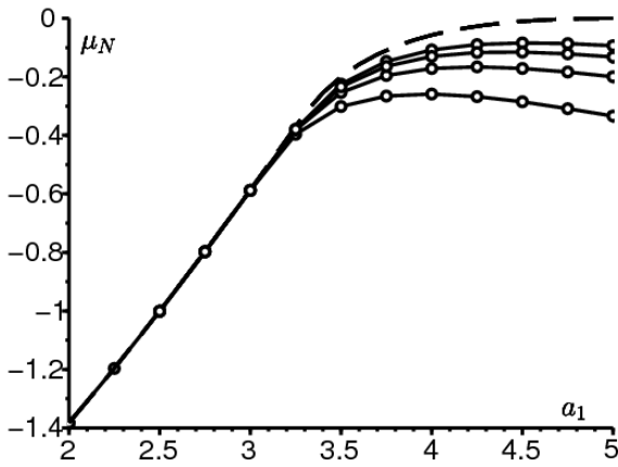
Рисунок 1. Пунктирная линия: \Lambda определяется формулой (3) как функция a_1 , Сплошные линии с точками: \mu_N для N = 10^3, 10^4, 10^5 и 10^6 (снизу вверх).
