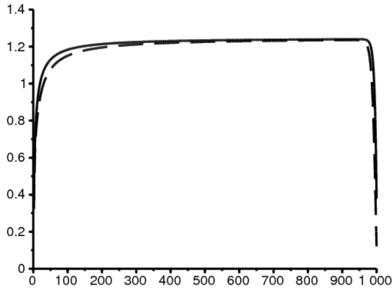
Рисунок 2. Корпус a_1 = 2,5 . Мы отслеживаем n^\beta(b/a_1)^n \pi_{n,1} (сплошная линия) и n^{\beta+1}(b/a_1)^n \pi_{n,2} k_1/h_2 (пунктирная линия) в зависимости от n . Используем усеченную матрицу \mathcal{M}^{(N)} с N = 1000 .
