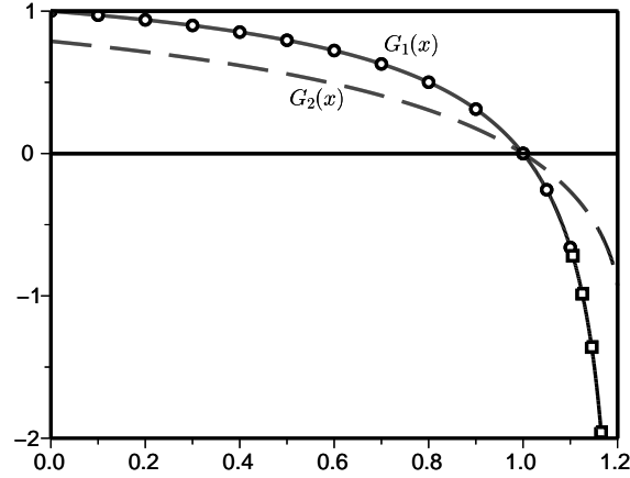
FIGURE 3 – Le cas où a_1 = 2,5 . Les fonctions génératrices G_1(x) (ligne continue) et G_2(x) (en pointillé) sont tracées en fonction de x et calculées en utilisant la matrice \mathcal{M}^{(N)} avec N = 4000 . Les formules (23) et (24) pour G_1(x) sont représentées par des petits cercles et carrés.
