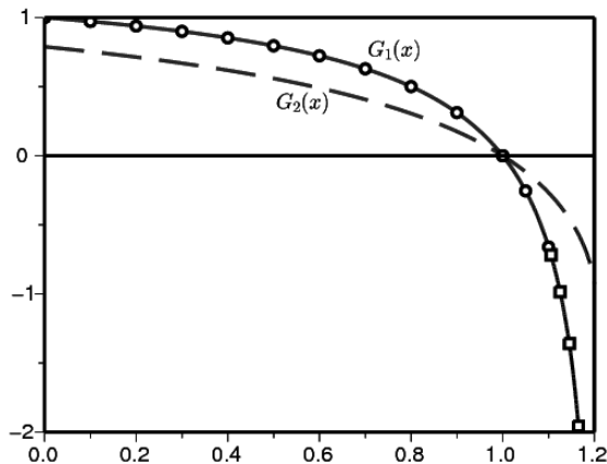
Abbildung 3. Der Fall a_1 = 2,5 . Wir verfolgen die generierenden Funktionen G_1(x) (durchgezogene Linie) und G_2(x) (gepunktete Linie) als Funktion von x . Man verwendet für die Berechnung die Matrix \mathcal{M}^{(N)} mit N = 4000 . Die Formeln (23) und (24) für G_1(x) werden durch kleine Kreise und Quadrate dargestellt.
