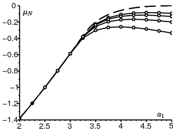
Abbildung 1. Gepunktete Linie: \Lambda gegeben durch Formel (3) als Funktion von a_1 . Durchgehende Linien mit Punkten: \mu_N für N = 10^3, 10^4, 10^5 und 10^6 (von unten nach oben).
