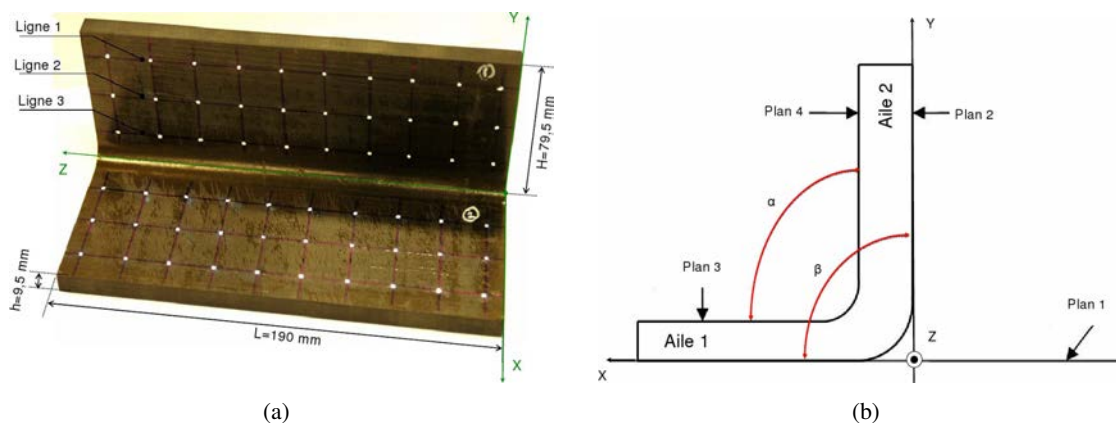
Figure 1 – (a) Points de de mesures d'épaisseur de la pièce en L, (b) désignation des angles et des plans.
