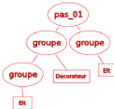
Figure 9 – Représentation du décorateur
