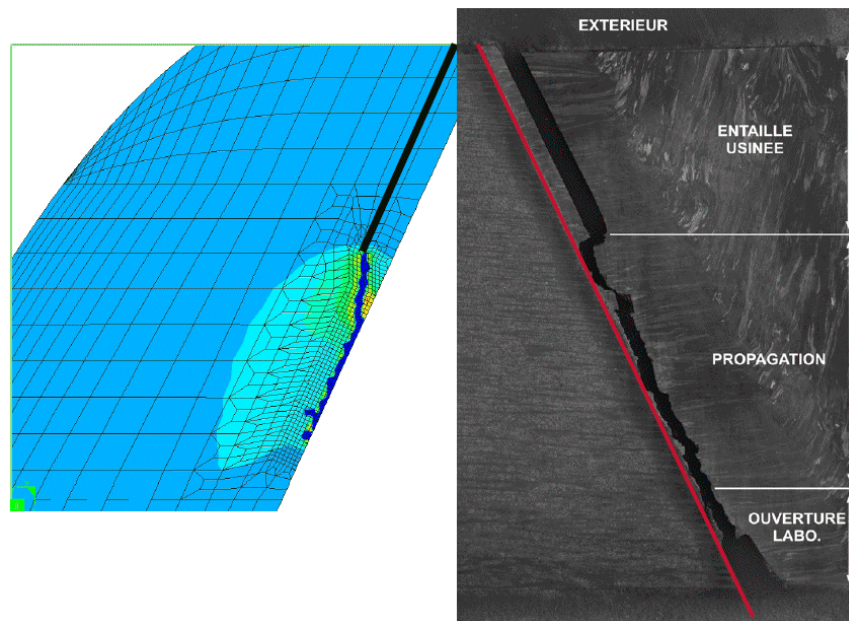
Figure 10 : Comparaison des chemins de fissuration calculés avec le modèle de Wilkins et observé sur la maquette ADIMEW [10]
