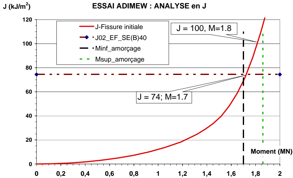
Figure 7 : Variation de J pour la fissure de la maquette ADIMEW et comparaison aux valeurs de J_{02} et de moments mesurés à l’amorçage
