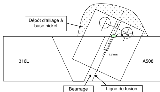
Figure 3 : Prélèvement d'éprouvette C(T) dans l'épaisseur de la liaison bimétallique
