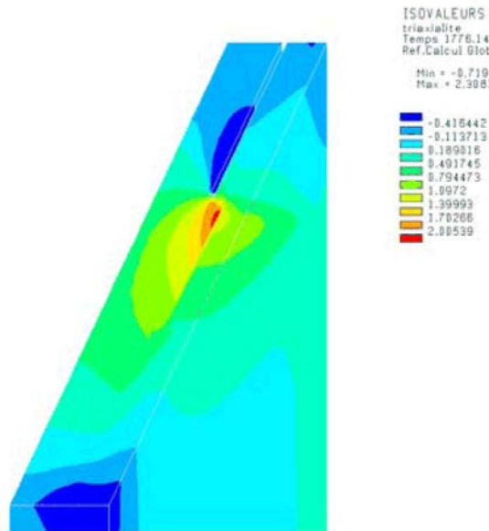
Figure 8 : Valeurs de la triaxialité des contraintes près de l’interface à l’amorçage
