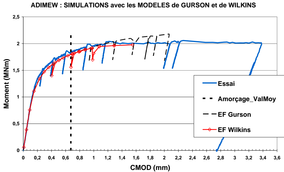
Figure 9 : Comparaison des chemins de fissuration calculés avec le modèle de Wilkins et celui observé sur la maquette ADIMEW [10]
