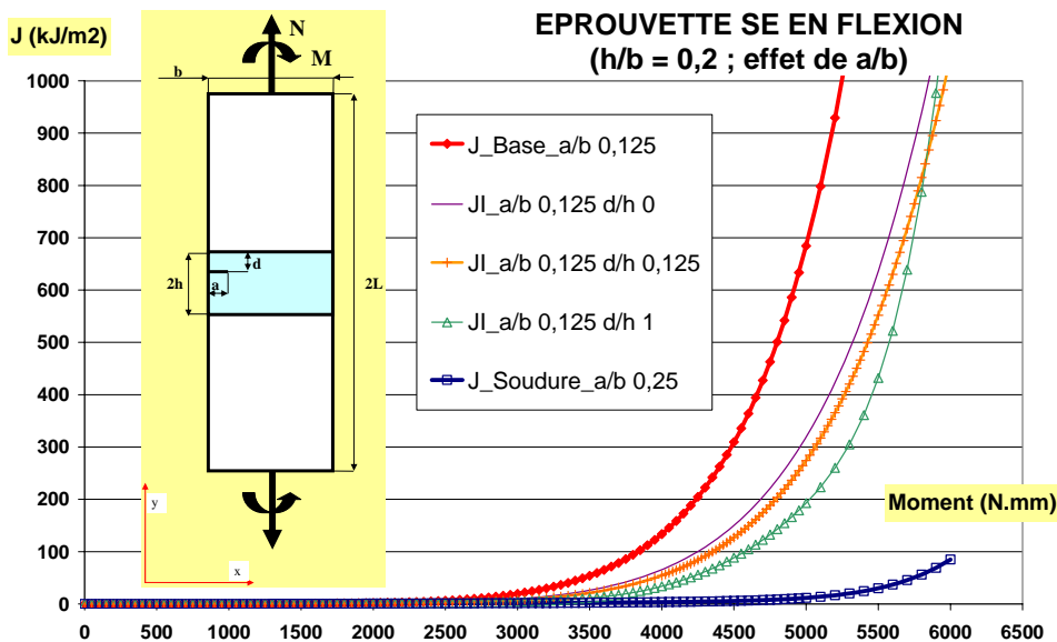
Figure 5 : Variation de J dans des éprouvette SE(B) à fissure égale à 1/8^{\text{ème}} de l'épaisseur pour les cas homogènes métal de base et joint soudé et pour des joints soudés comportant une fissure centrée, proche de l'interface ou à l'interface ( M_y = 2,3 )
