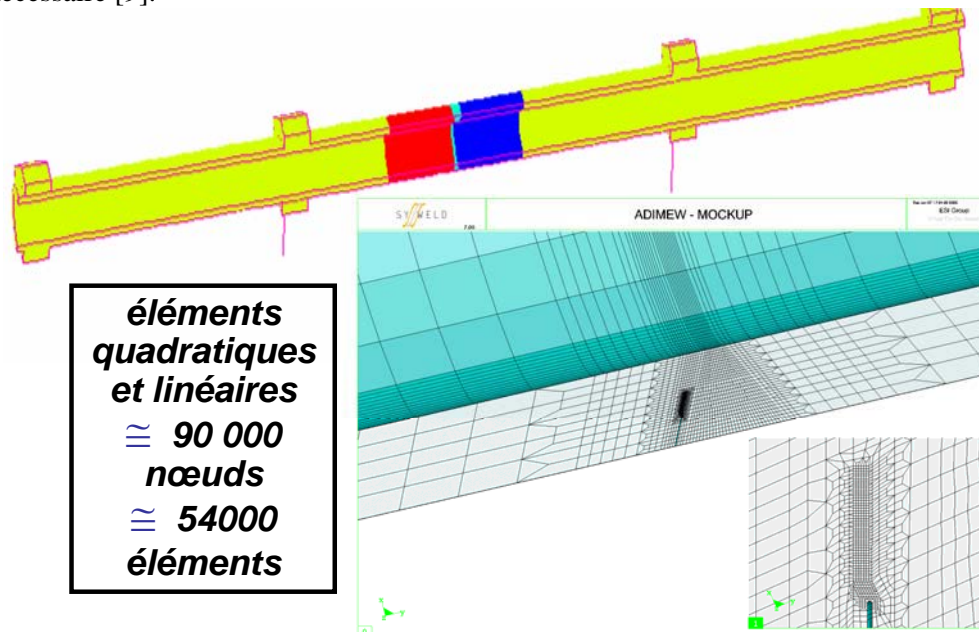
Figure 6 : Maillage d'un demi-modèle de la maquette ADIMEW
