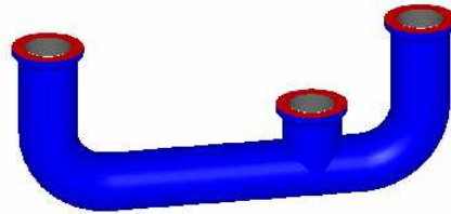
Figure 10 – Modélisation solide : en rouge les bases des tuyaux encastrés, en gris la paroi interne du tuyau où est affectée la pression du fluide
