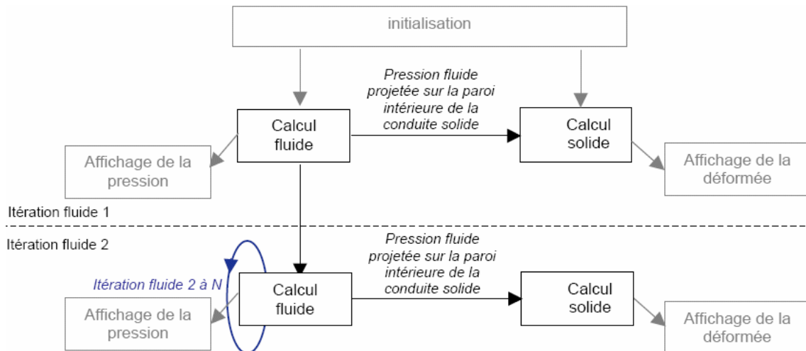
Figure 13 – Schéma de chaînage
