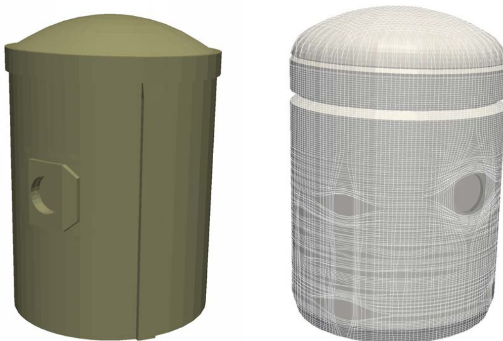
Figure 2 – CAO de l'enceinte et du ferrailage.
