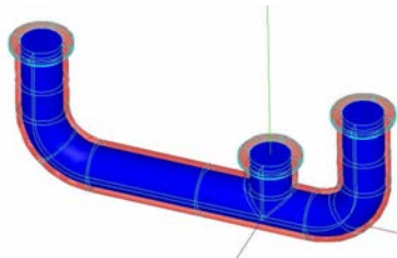
Figure 6 – Té de mélange : partie solide en rouge et écoulement fluide en bleu
