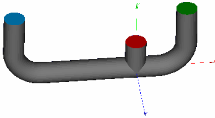
Figure 9 – Modélisation fluide : en bleu, une entrée froide, en rouge une entrée chaude, en vert une sortie et en gris la paroi.
