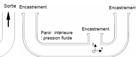
Figure 8 – Conditions aux limites pour le solide
