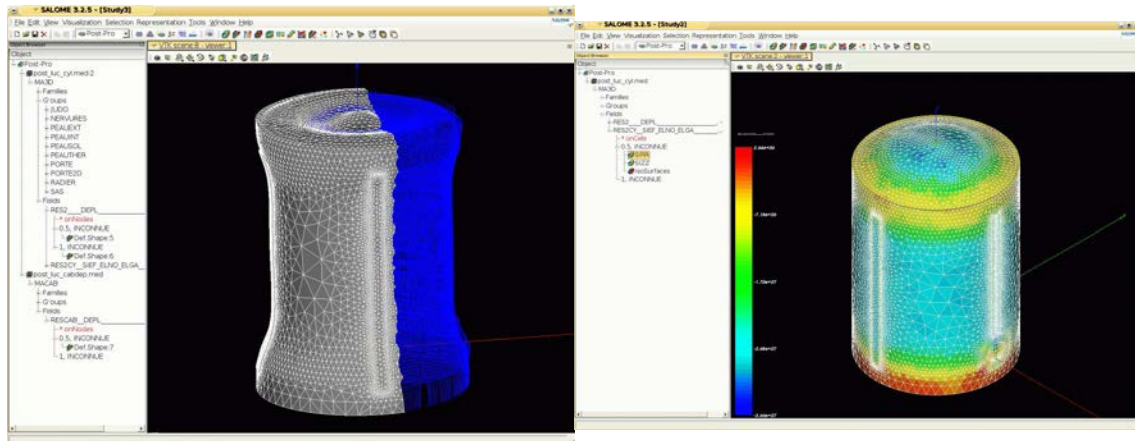
Figure 5 – Visualisation de la déformée et de la contrainte \sigma_{rr} .
