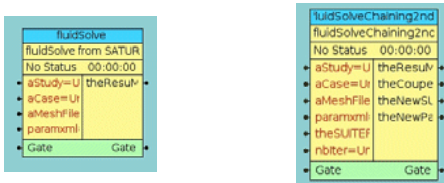
Figure 14 – Nœuds de calcul du superviseur de Salome-Meca pour Code_Saturne
