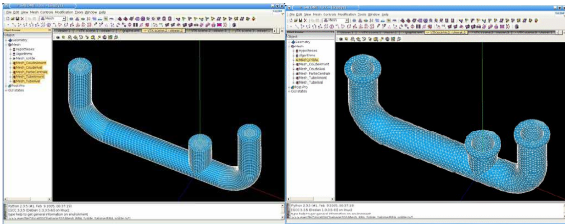
Figure 11 – Maillage de la partie fluide en hexaèdres
