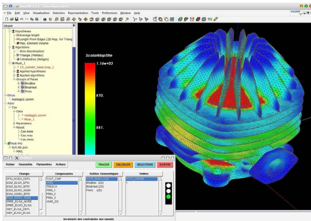
Figure 1 – Salome-Meca : visualisation de la contrainte de Von Mises.
