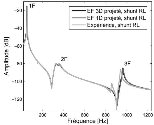
Figure 2 – FRF observée en bout de poutre
