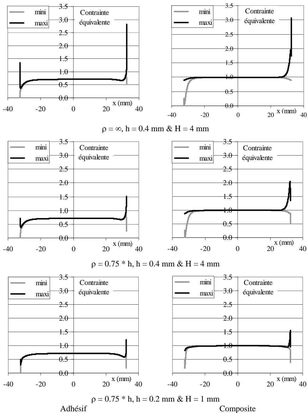
Figure 2 – Evolution suivant l’abscisse des valeurs extrémales des contraintes équivalentes normalisées dans la colle et dans le composite pour des substrats sans bec ( d = 0 ) et pour D = 0 et pour une sollicitation de traction-cisaillement.
