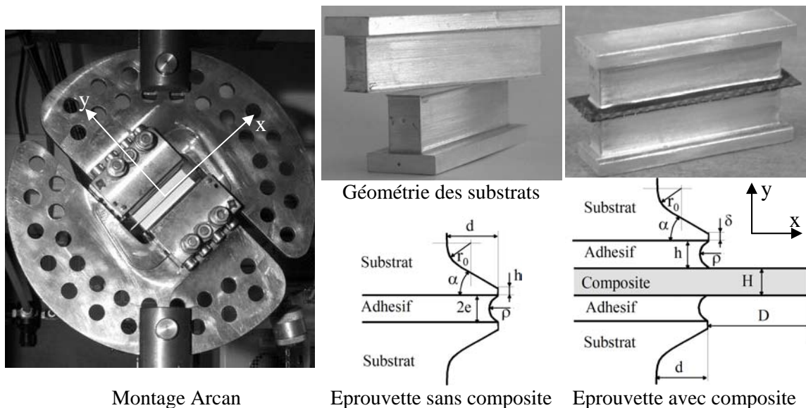
Figure 1 – Présentation du montage Arcan et des éprouvettes utilisées
