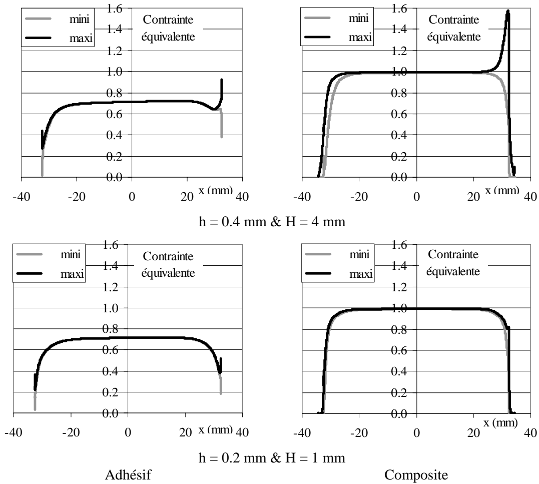
Figure 3 – Evolution suivant l'abscisse des valeurs extrémales des contraintes équivalentes normalisées dans la colle et dans le composite pour des substrats avec bec et pour une sollicitation de traction-cisaillement.
