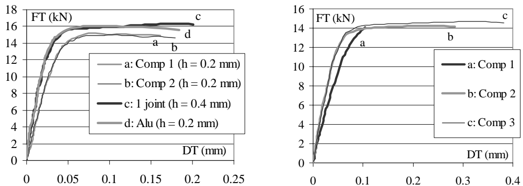
a - Composites unidirectionnels b - Composites multidirectionnels (h=0.4mm) Figure 4 – Résultats expérimentaux pour des sollicitations de traction-cisaillement
