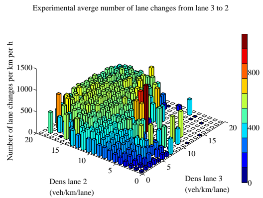
(d) lane 3 to 2
