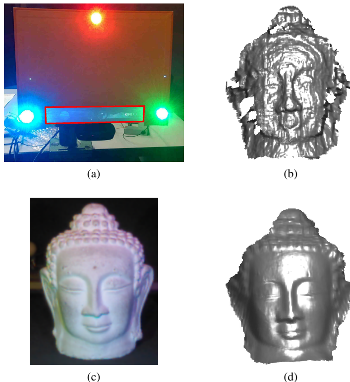
FIGURE 1. (a) Photographie de notre montage, prise depuis la scène à reconstruire : un capteur RVB-D (encadré en rouge) est équipé de trois LEDs colorées en rouge, vert et bleu. (b) Rééclairage de la reconstruction 3D fournie par le capteur de profondeur, qui est bruitée et comporte des données manquantes. (c) Image RVB fournie par ce montage, qui nous permet d'appliquer la stéréophotométrie colorée. (d) Rééclairage du résultat de la fusion de données RVB-D par l'approche proposée.
