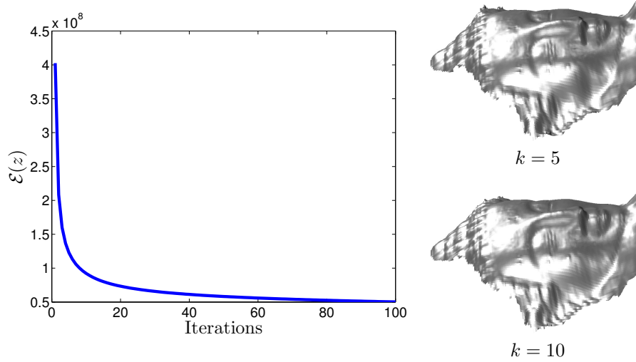
FIGURE 4. À gauche : graphe de l'énergie \mathcal{E}(z) définie en (44), en fonction des itérations, pour \lambda_0 = 10^4 . Malgré l'absence de garantie sur la convergence du schéma de résolution proposé, nous observons expérimentalement que \mathcal{E}(z) décroît au cours des itérations. À droite : relief estimé après k itérations. Même si la convergence du schéma vers la solution de (44) est plutôt lente, 5 à 10 itérations ( \approx 2 s de calcul sur un processeur I7 récent, avec des codes Matlab non optimisés) suffisent en pratique à obtenir un résultat qualitativement satisfaisant.
