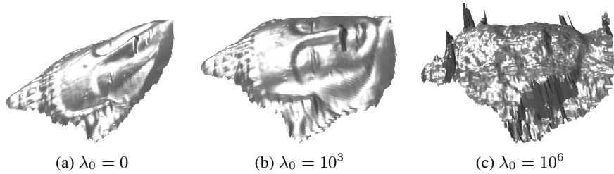
FIGURE 5. Reconstructions 3D obtenues pour différentes valeurs du paramètre \lambda_0 . (a) Contrairement aux cas où m > 3 images RVB sont disponibles (cf. figure 3), la stéréophotométrie à une seule image RVB comporte un biais. (b) Ce biais disparaît lorsque \lambda_0 augmente. (c) Toutefois, le relief obtenu avec une valeur trop élevée de \lambda_0 est similaire au relief très bruité fourni par le capteur RVB-D (cf. figure 6-a).
