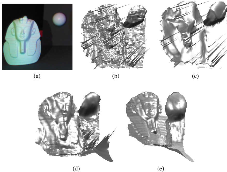
FIGURE 7. (a) Exemple d'image RVB obtenue avec notre montage (cf. figure 1-a). (b) Fonction de profondeur z_0 associée. (c) Fusion de données RVB-D par shape-from-shading non calibré (Or-el et al., 2015) : le relief est sur-lissé. (d) Fusion de données RVB-D par l'approche L^2 - L^2 : les discontinuités de profondeur induisent des artefacts, (e) qui sont fortement atténués en utilisant l'approche robuste L^1 - L^1 .
