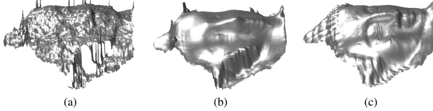
FIGURE 6. (a) Relief z_0 fourni par le capteur RVB-D. (b) Fusion de données RVB-D par shape-from-shading non calibré (Or-el et al., 2015). (c) Reconstruction 3D L^2 - L^2 obtenue pour \lambda = 10^4 , valeur qui donne visuellement le meilleur résultat.
