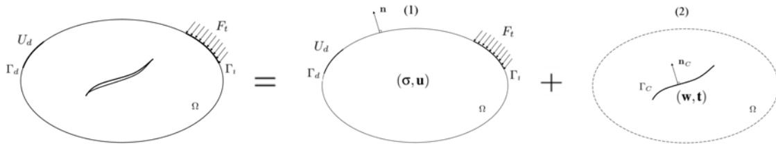
Figure 1 – Problème de fissuration découpé en un problème structure global (1) et un problème d'interface local (2).
