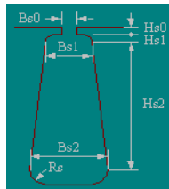
Fig. 5. Slot type
