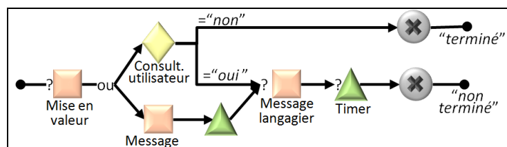
Fig. 12. aLDEAS : patron d'étape de pas-à-pas guidé
