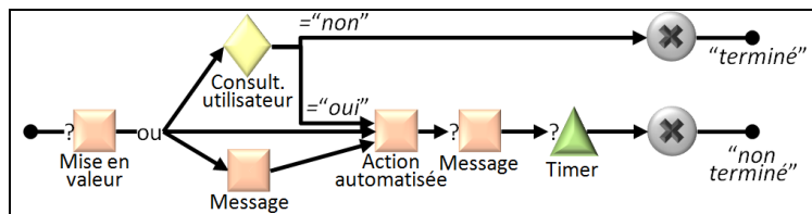
Fig. 11. aLDEAS : patron d'étape de pas-à-pas automatisé
