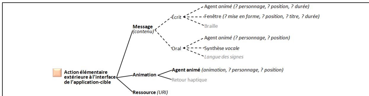
Fig. 6. aLDEAS : actions d'assistance élémentaires extérieures à l'application-cible
