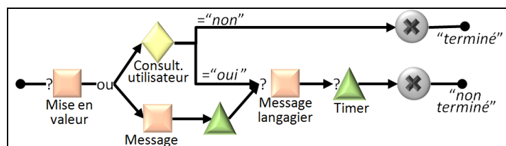
Fig. 12. aLDEAS : patron d'étape de pas-à-pas guidé
