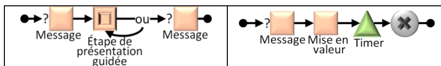
Fig. 16. Patron d’étape de présentation guidée
