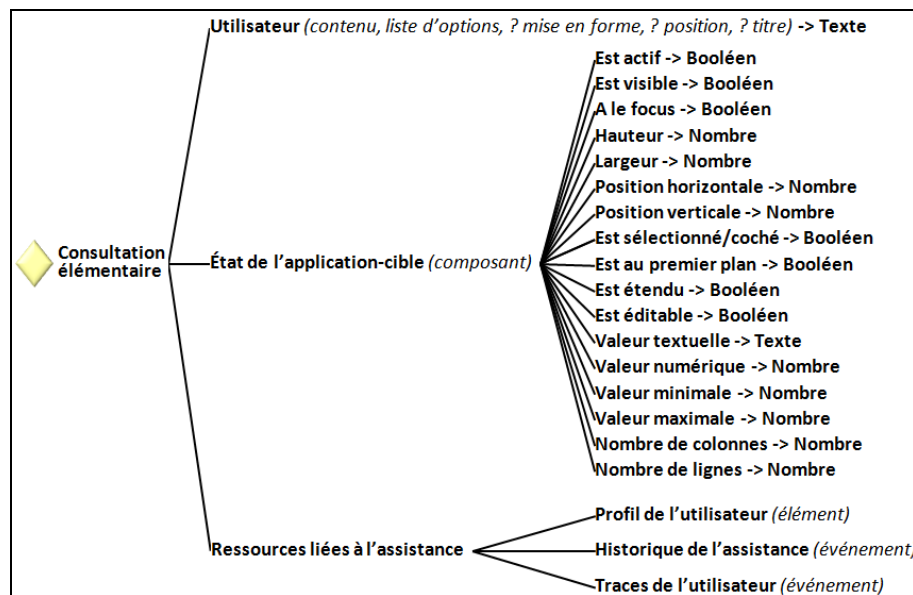
Fig. 4. aLDEAS : consultations élémentaires
