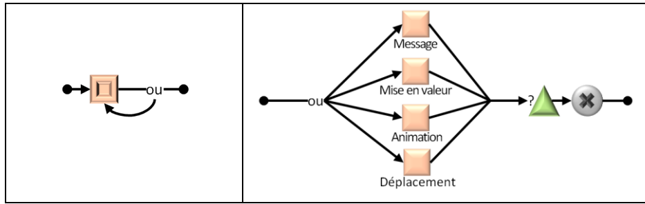
Fig. 20. aLDEAS : patron d'action d'agent animé
