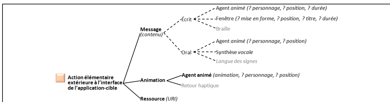
Fig. 6. aLDEAS : actions d'assistance élémentaires extérieures à l'application-cible
