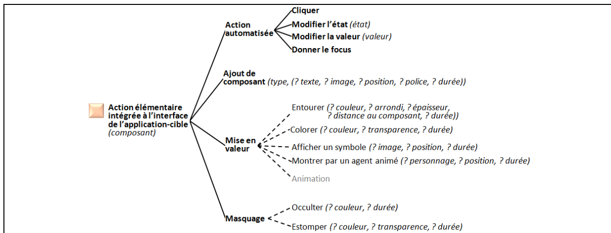
Fig. 5. aLDEAS : actions d'assistance élémentaires intégrées à l'application-cible
