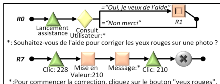
Fig. 9. Exemple des règles d'assistance R0 et R7 pour PhotoScape
