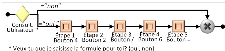
Fig. 13. Exemple de pas-à-pas automatisé pour la calculatrice
