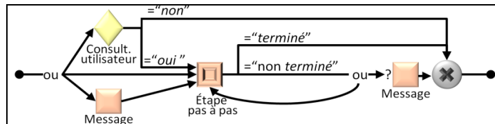
Fig. 10. aLDEAS : patron de pas-à-pas
