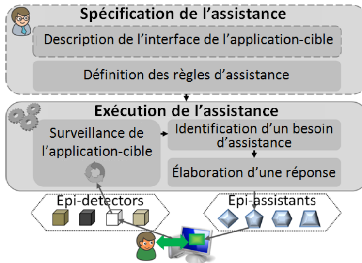
Fig. 1. Processus d'adjonction d'un système d'assistance épiphyte à une application existante
