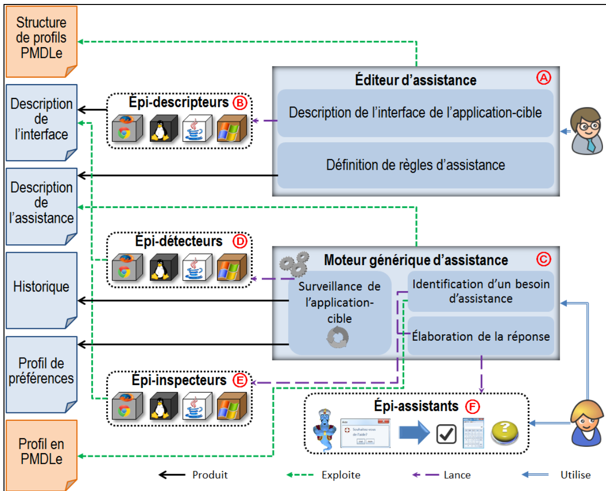
Fig. 23. Architecture de SEPIA
