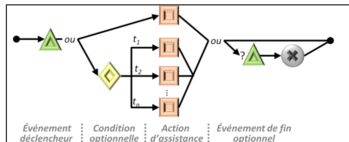
Fig. 8. Patron de règles d'assistance
