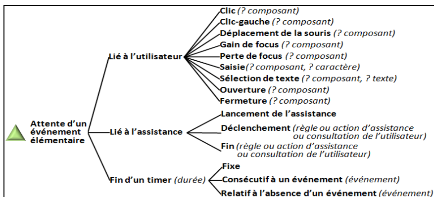
Fig. 3. aLDEAS : attentes d'événements élémentaires
