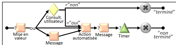
Fig. 11. aLDEAS : patron d'étape de pas-à-pas automatisé
