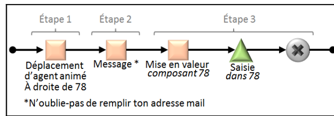
Fig. 22. Exemple d'action d'agent animé pour un formulaire d'inscription
