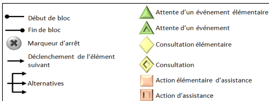
Fig. 2. Composants d'aLDEAS
