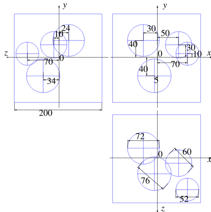
FIGURE 6 – Dimension du modèle emmental en mm
