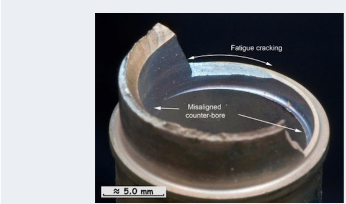
Figure: Fissuration de la turbine du réacteur
