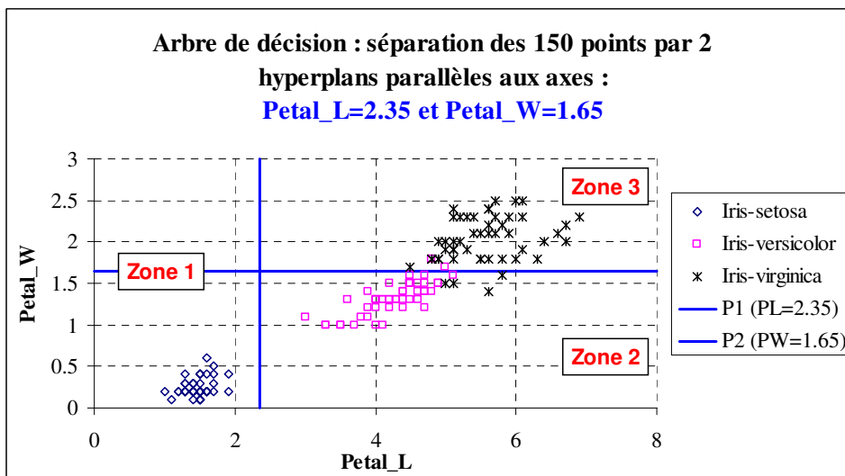
FIG. 4 – Résultat sur les 150 iris d'un arbre de décision entraîné une fois sur 75 iris tirés au hasard (25 par classe) : 2 hyperplans séparateurs et 6 erreurs (2 pour la partie apprentissage et 4 pour l'autre).
